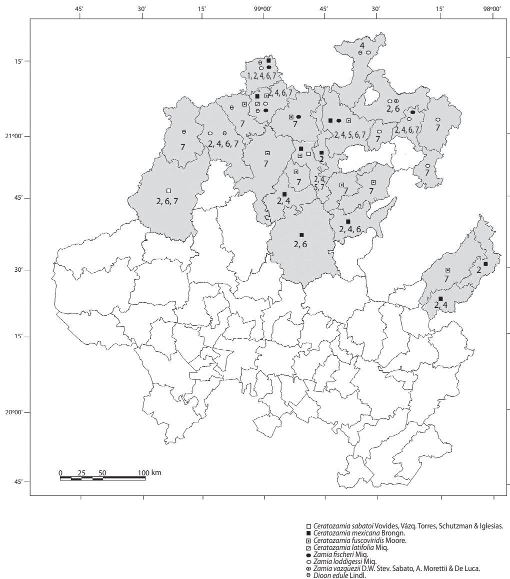
Fig. 2. Distribución de las especies de cícadas presentes en los municipios del estado de Hidalgo. Los números indican la fuente de donde se obtuvo la información: 1. Contreras et al. 2001, 2. Contreras et al. 2003, 3. Yáñez 2006, 4. Mejenes et al. 2007, 5. Osborne et al. 2006, 6. Ejemplares de herbarios (MEXU, IEB, FCME, ENCB, HGOM), 7. Recolectas botánicas (Aurelia Vite Reyes, María T. Pulido y Juan C. Flores-Vázquez).
