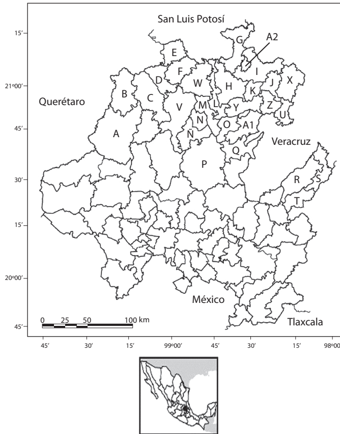
Fig. 1. Municipios del estado de Hidalgo con presencia de cícadas: Zimapán (A), Pacula (B), Jacalade Ledezma (C), La Misión (D), Pisaflores (E), Chapulhuacán (F), San Felipe Orizatlán (G), Tlanchinol (H), Huejutla de Reyes (I), Atlapexco (J), Huazalingo (K), Lolotla (L), Molango de Escamilla (M), Juárez Hidalgo (N), Eloxochitlán (Ñ), Xochicoatlán (O), Metztlán (P), Zacualtipán de Ángeles (Q), San Bartolo Tutotepec (R), Huehuetla (S), Tenango de Doria (T), Xochiatipan (U), Tlahuiltepa (V), Tepehuacán de Guerrero (W), Huautla (X), Tianguistengo (A1). Municipios que faltan por muestrear: Calnali (Y), Yahualica (Z), Jaltocán (A2).
