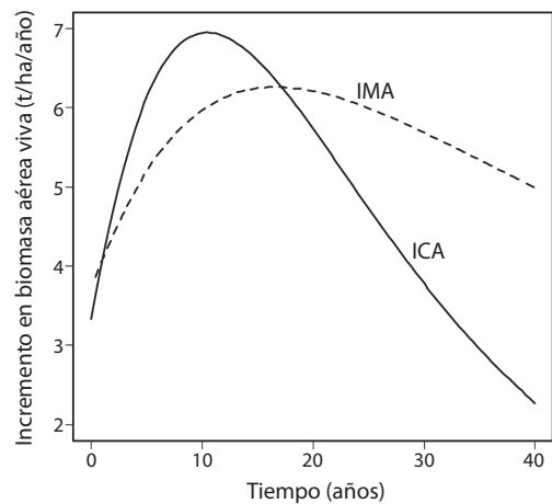
Fig. 3. Tasas absolutas de crecimiento o incremento corriente anual (ICA) y tasas medias de crecimiento o incremento medio anual (IMA) de la biomasa aérea viva (Bav) derivadas de la curva de rendimiento.
