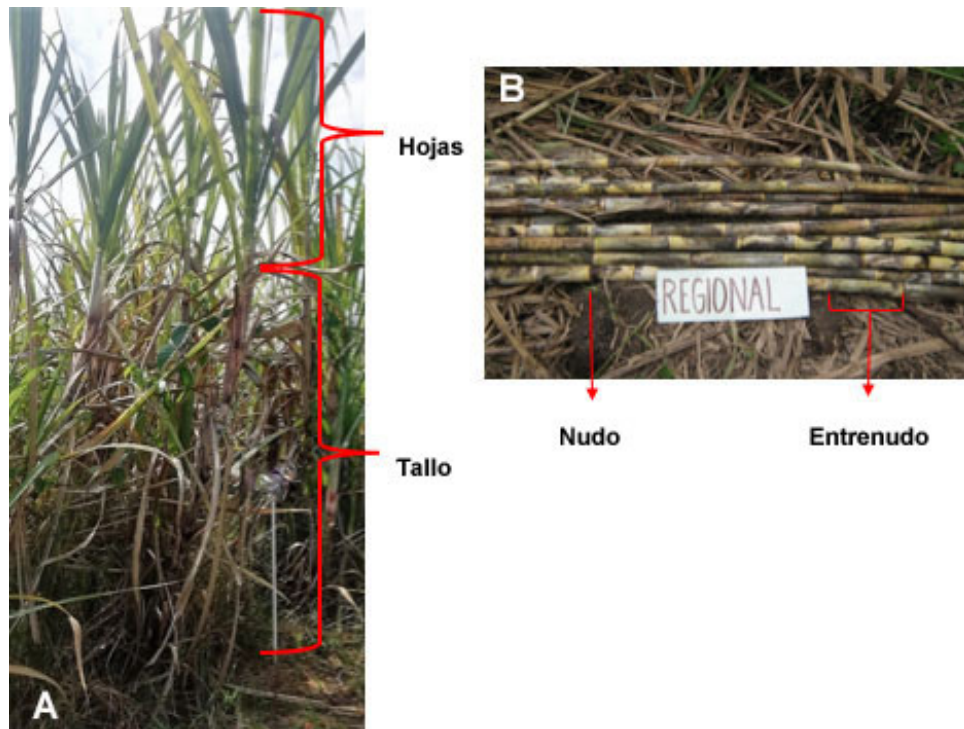
Figura 1. Variedad de caña de azúcar para panela Canal Point (CP 782018). A. Partes aéreas (tallo y hojas). B. Partes del tallo en caña de azúcar (entrenudo y nudo). Nariño, Colombia. 2008-2009.
