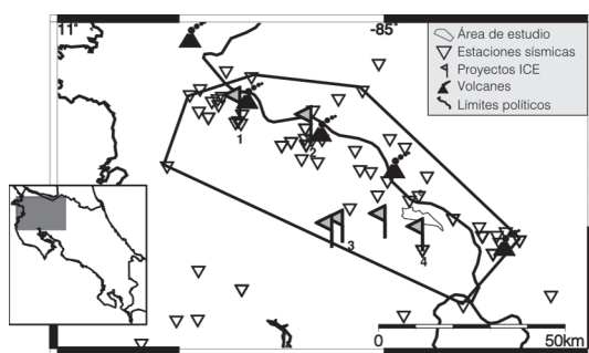
Fig. 1: Mapa de ubicación del área de estudio, estaciones sísmicas y proyectos del ICE. Símbolos numerados corresponden con los siguientes proyectos ICE: 1. Centro de Producción Pailas, 2. Centro de Producción Miravalles 3. Centros de Producción ARCOSA.
