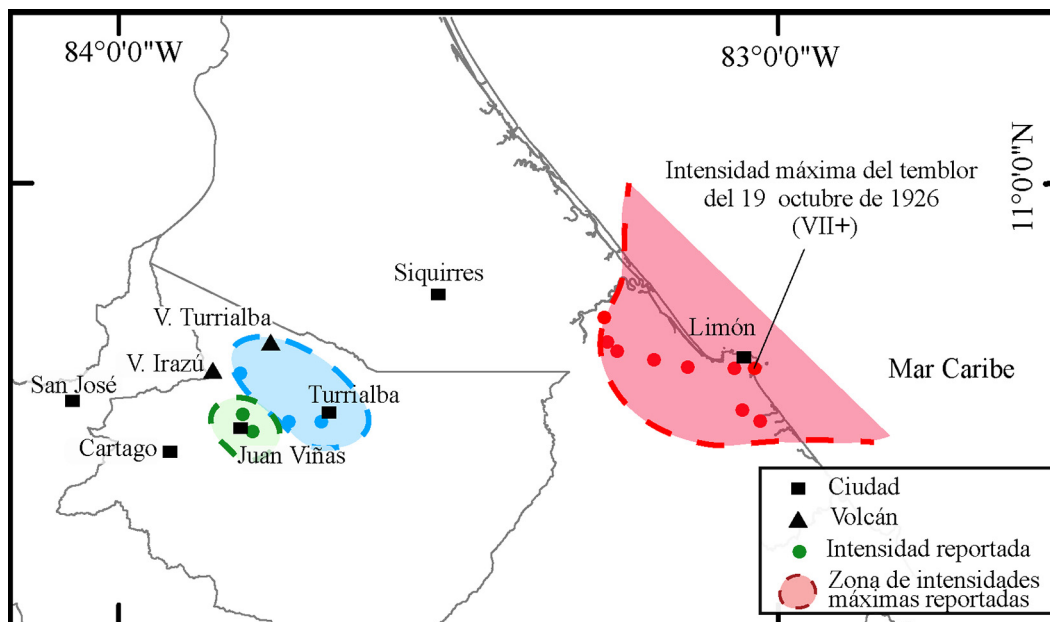
Fig. 1: Áreas de percepción de máximas intensidades para las secuencias sísmicas de junio y agosto de 1913 (en verde), abril de 1920 (en azul), y los sismos de 1926 y 1953 (en rojo). El área de máxima intensidad para el sismo del 7 de enero de 1953 está basado en Boschini (1989).
