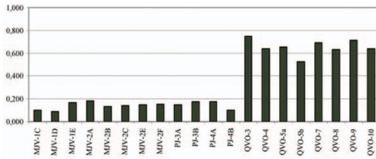
Fig. 3: Comportamiento del índice de aplastamiento (IA) de las partículas de Au en los depósitos de placeres marinos costeros de las playas Mejías (MJV) y Jiguani (PJ). A manera de comparación también se muestra el IA de los granos de oro los depósitos fluviales del río Quesigua (QVO).
