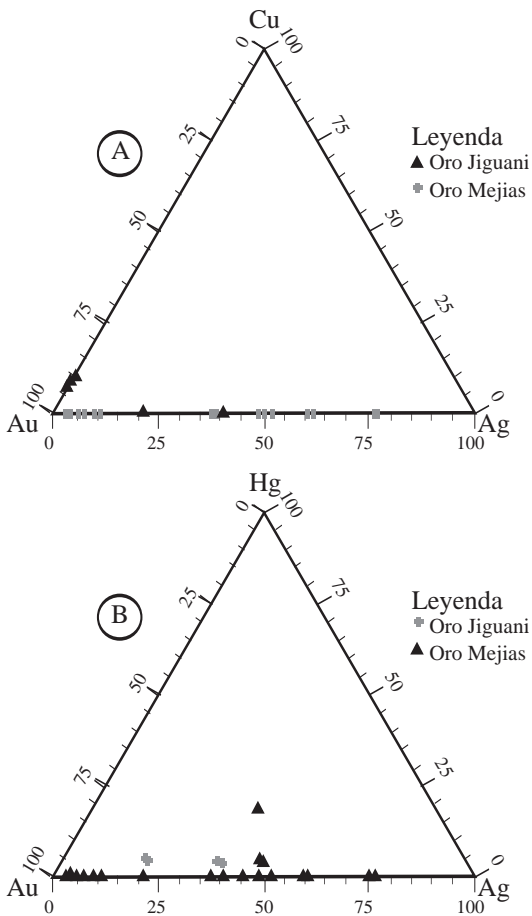
Fig. 5: Composición química de las partículas de oro estudiadas en los sistemas Au-Ag-Cu (A) y Au-Ag-Hg (B).
