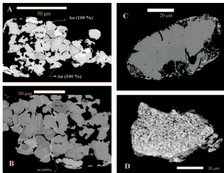
Fig. 4: Imágenes de electrones retrodispersados de partículas de oro de composición compleja de los placeres Mejías (ABC) y Jiguani (D). Nótese el aspecto corroído de los bordes y superficies de las partículas, así como granos de oro de diferentes composiciones. Las zonas más claras corresponden a las mayores concentraciones de Au.
