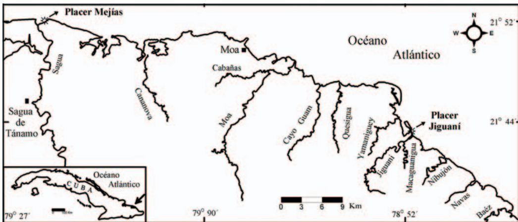
Fig. 1: Mapa de ubicación de la región de estudio, noreste de Cuba oriental.
