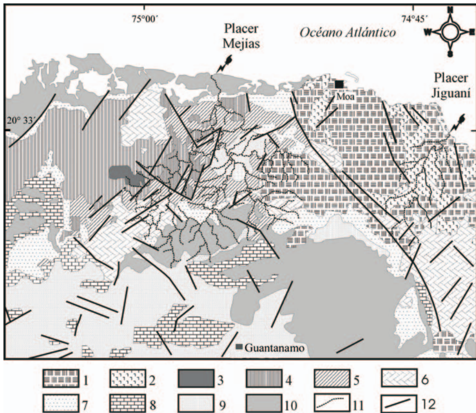
Fig. 2: Mapa geológico de la región estudiada: 1) Macizo ofiolítico Moa-Baracoa (constituido por peridotitas, principalmente harzburgitas); 2) Gabros del complejo de acumulados máficos; 3) Complejo metamórfico "La Coreá" (anfíbolitas, plagiogneis); 4) Macizo ofiolítico Mayarí-Cristal (constituido por peridotitas, principalmente harzburgitas y dunitas); 5) Materiales sedimentarios detríticos asociados a las cuencas transportadas ( piggy back ) del Campaniense tardío al Daniense; 6) Rocas volcánicas y volcanosedimentarias del arco de islas volcánico del Cretácico; 7) Rocas volcánicas y volcanosedimentarias del arco de islas volcánico del Paleógeno. Cuencas transportadas ( piggy back ) del Eoceno Medio al Superior (Oligoceno?); 8) Formaciones carbonatadas; 9) Molasa flyschoid. Cobertura Neógena-Cuaternaria; 10) Calizas, gravas, arenas, arcillas; 11) Red Fluvial; 12) Fallas.
