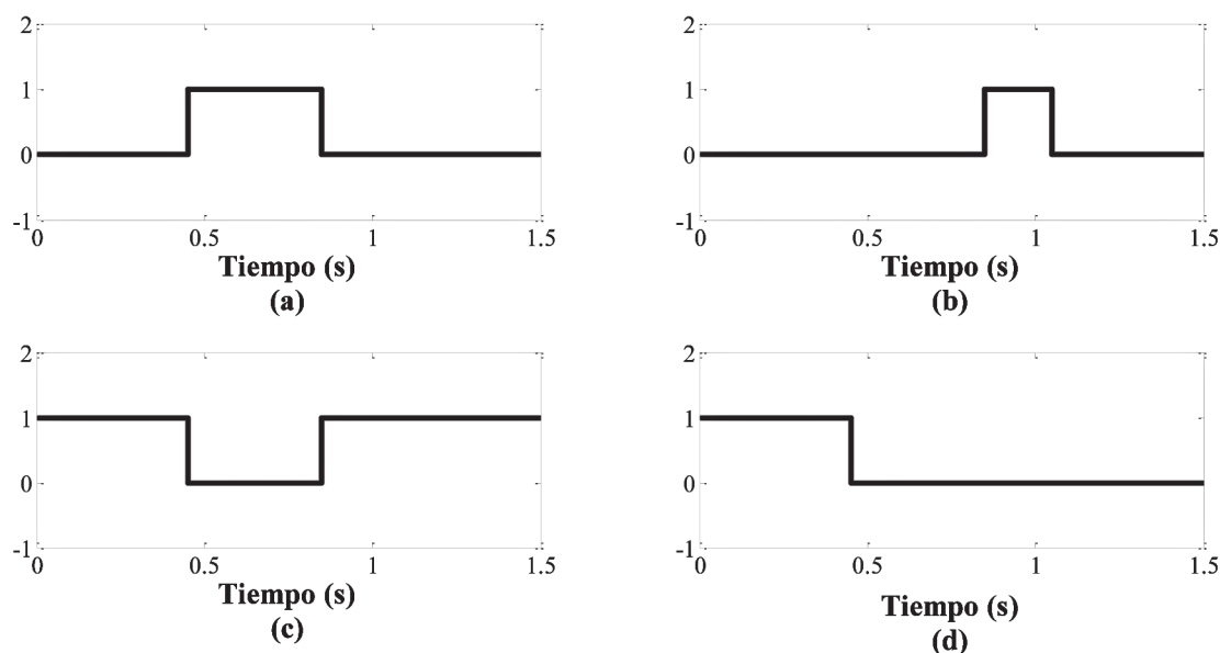
Figura 5. Señales lógicas cuando el interruptor 152L opera normalmente (a) falla simulada, (b) señal de auto-recierre, (c) posición del interruptor 152L, (d) posición del interruptor 152M.
