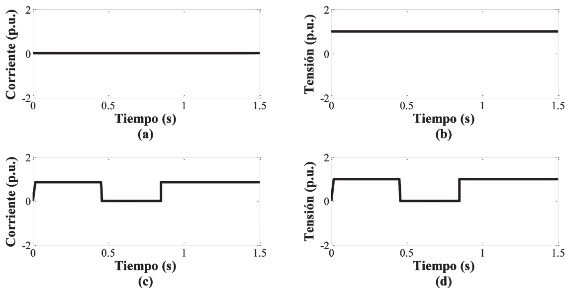
Figura 8. Señales lógicas cuando el interruptor 152L está en mantenimiento (a) flujo de corriente a través de 152L, (b) tensión eléctrica en la Barra A, (c) flujo de corriente a través de 152M, (d) tensión eléctrica en el interruptor 152M.
