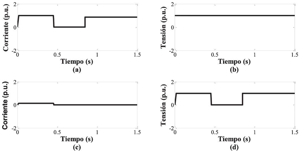
Figura 6. Flujos de corriente y tensiones eléctricas durante la operación normal (a) flujo de corriente a través de 152L, (b) tensión eléctrica en la Barra A, (c) flujo de corriente a través de 152M, (d) tensión eléctrica en el interruptor 152M.
