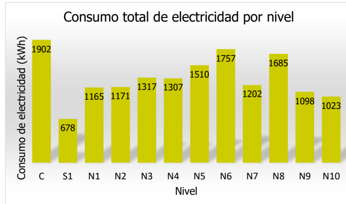
Fig. 4. Consumo total de electricidad por nivel de TLL.
