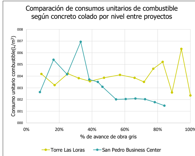
Fig. 13. Comparación de consumos unitarios de combustible según cantidad de concreto por nivel entre TLL y SPBC.
