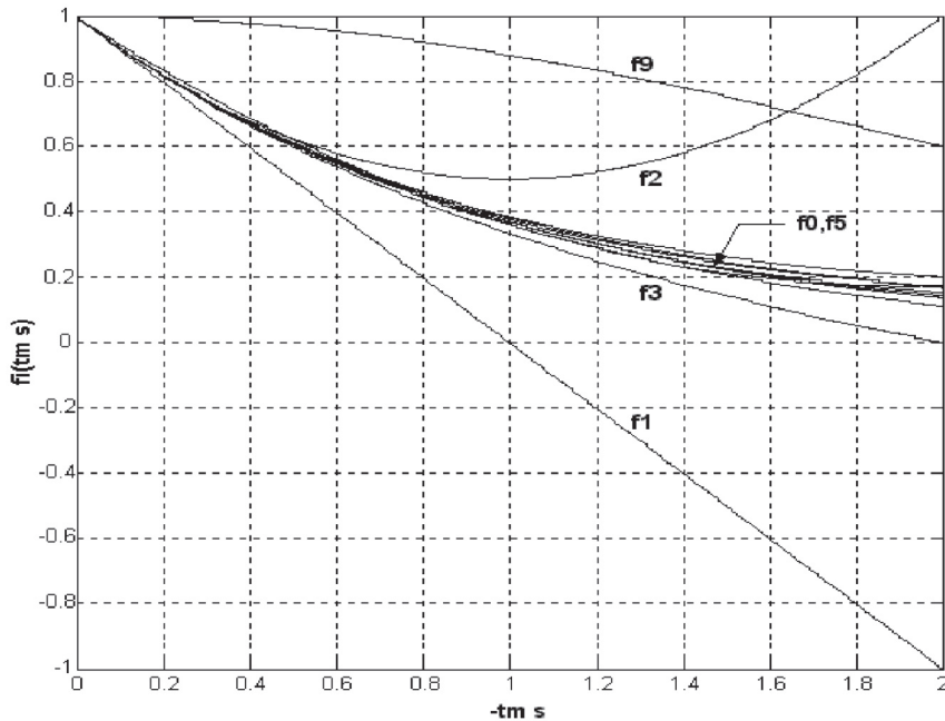
Figura 2. Aproximaciones de la función exponencial
