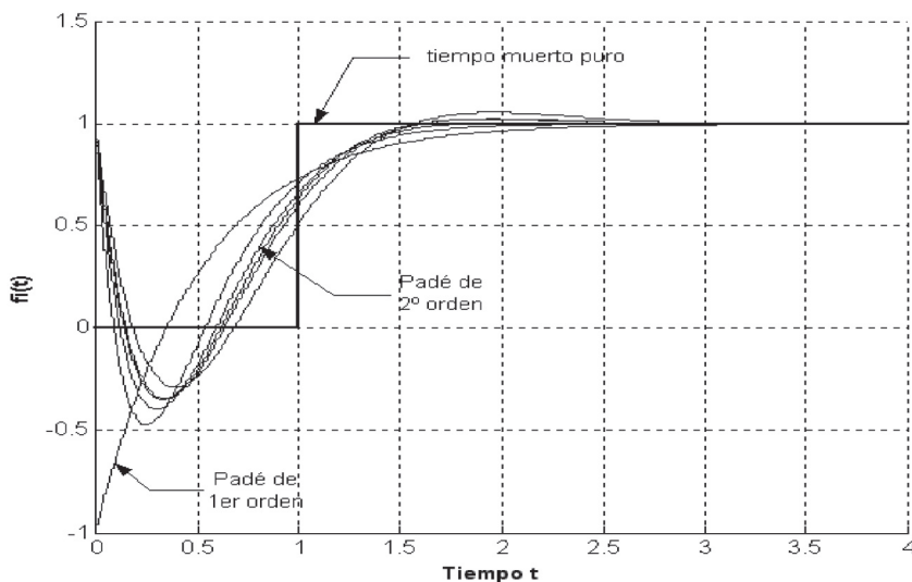
Figura 3. Respuesta a un escalón unitario, t_m=1
