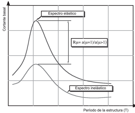
Figura 5. Obtención de factores de reducción por ductilidad mediante la relación de ordenadas Fuente: (Vielma, 2003)
