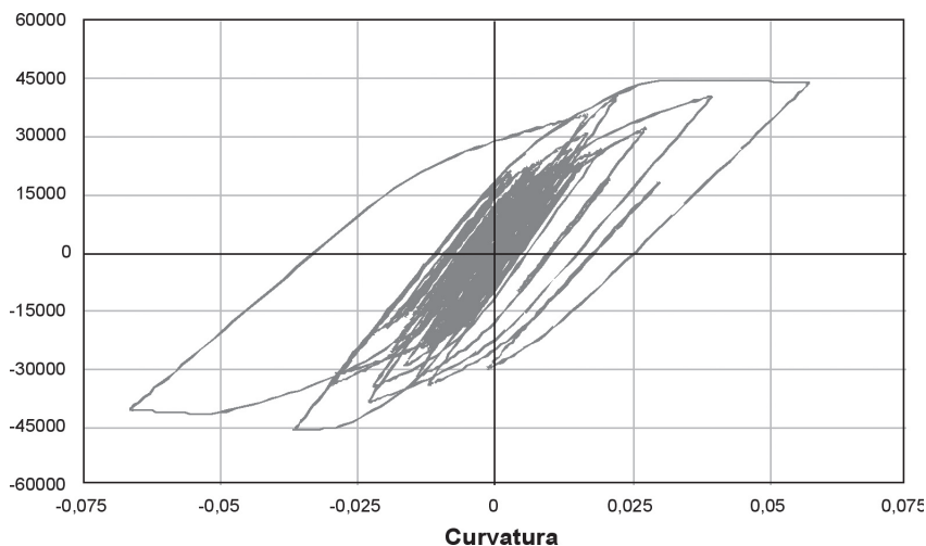
Figura 4. Respuesta histerética de pórtico de acero.
