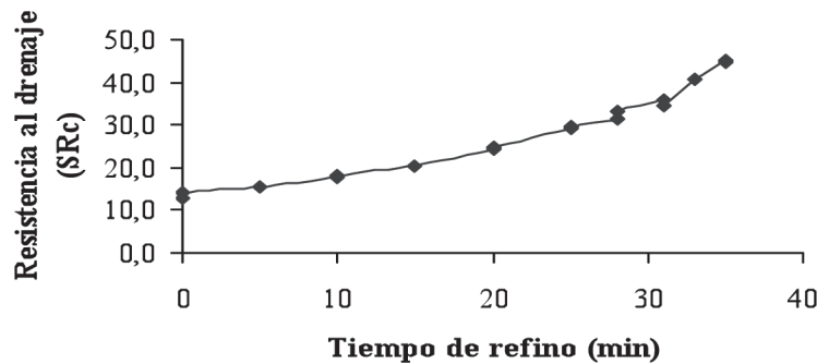
Figura 2. Curva de refinado en la pila holandesa de la mejor pulpa obtenida con el pulpeo soda-antraquinona.
