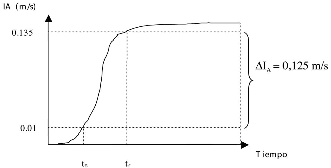
Figura 4. Gráfico de Husid y límites para la determinación de la duración efectiva. t_c es donde se alcanza una I_A de 0,01 m/s, t_f corresponde a una I_A de 0,135 m/s, o sea, a una energía acumulada de 0,125 m/s. Fuente: (Bommer & Martínez, 1999).
