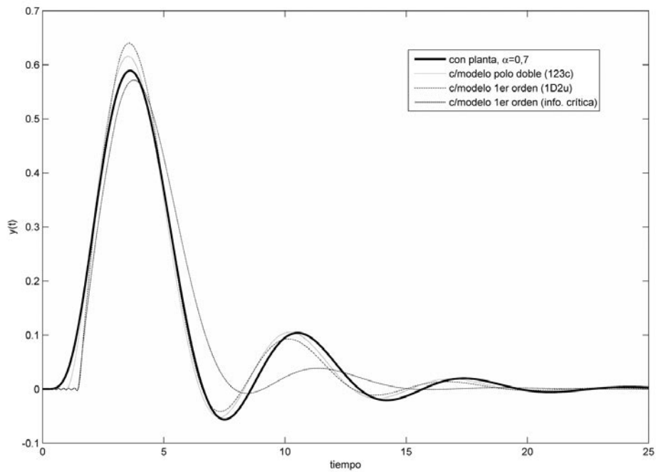
Figura 2. Comparación de las respuestas del control regulador, planta con \alpha = 0,70 . Fuente: (El autor)
