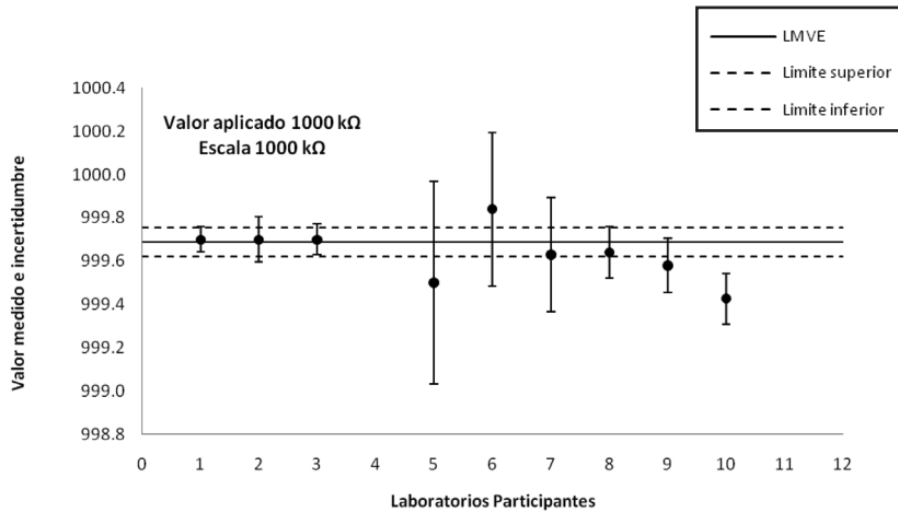
Figura 16. Gráfico de resultados de la comparación en 1000 kΩ.
