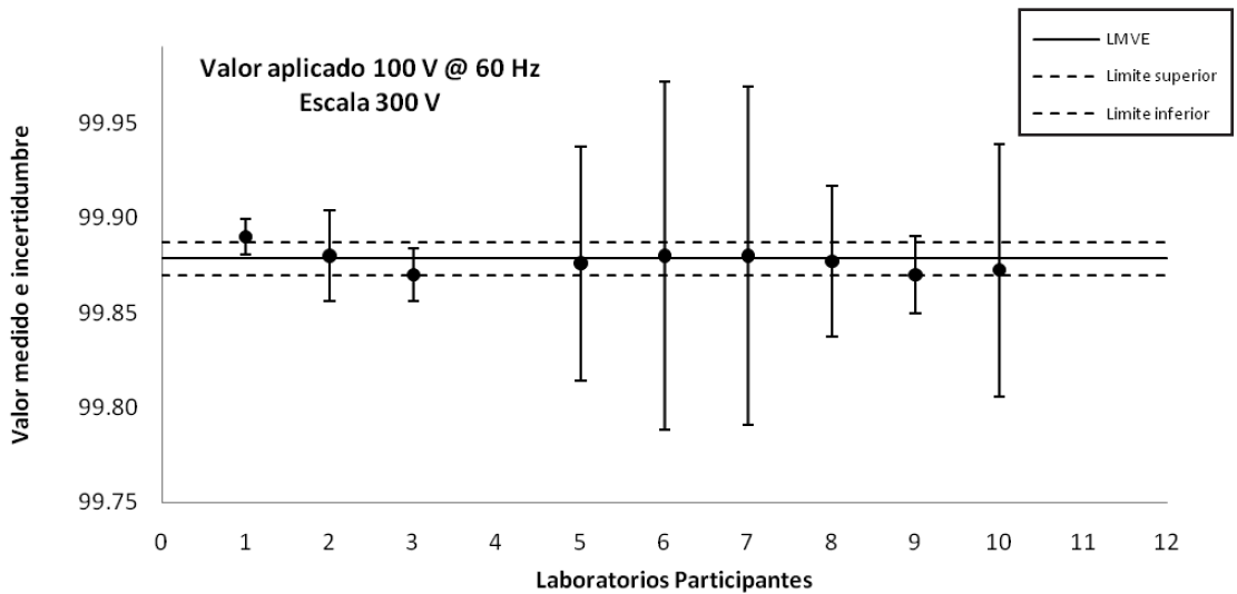
Figura 6. Gráfico de resultados de la comparación en 100 VCA @ 60 Hz. Fuente: (LMVE, 2009).
