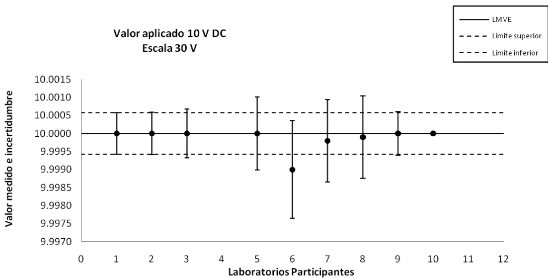
Figura 3. Gráfico de resultados de la comparación en 10 V.
