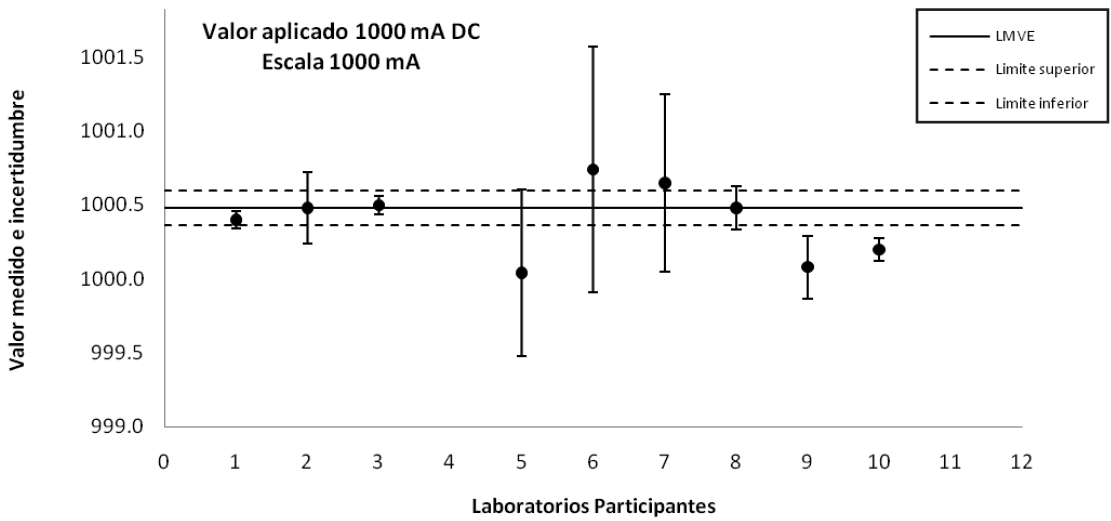
Figura 5. Gráfico de resultados de la comparación en 1000 mA DC. Fuente: (LMVE, 2009).
