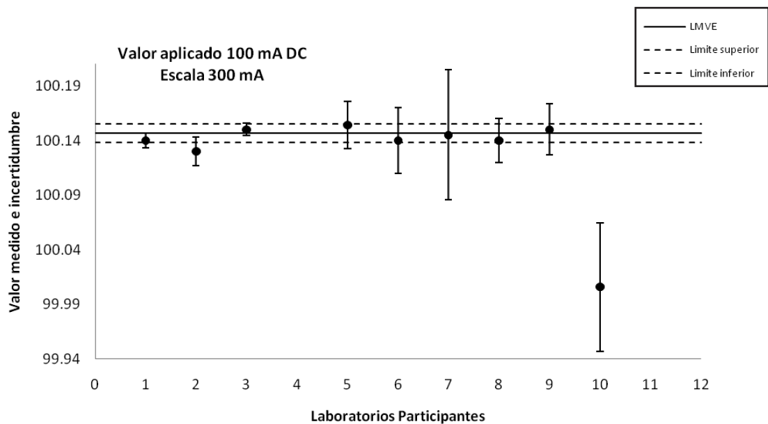
Figura 4. Gráfico de resultados de la comparación en 100 mA DC.
