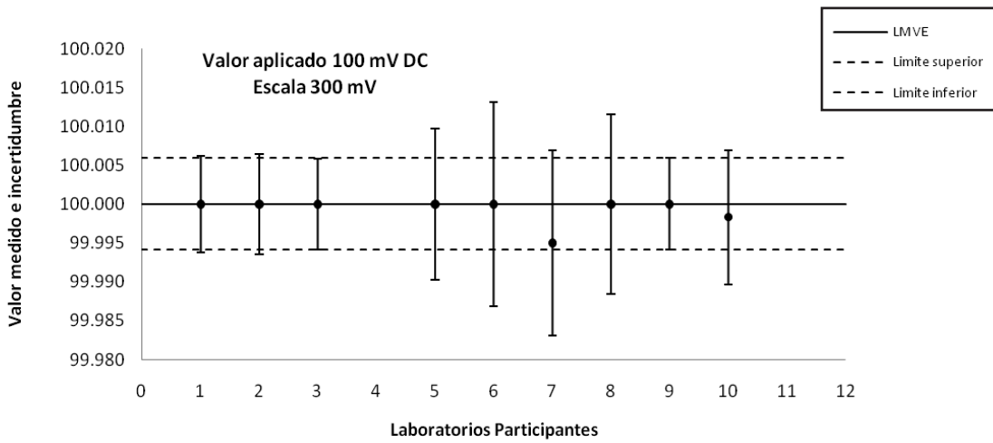
Figura 1. Gráfico de resultados de la comparación en 100 mV. Fuente: (LMVE, 2009)
