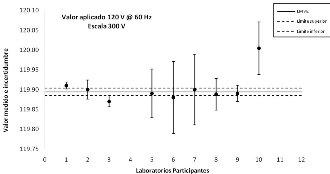
Figura 7. Gráfico de resultados de la comparación en 120 VCA @ 60 Hz.
