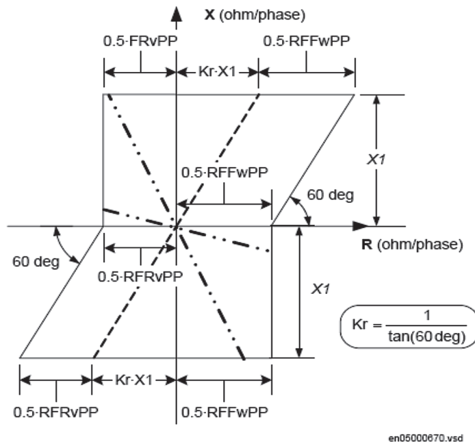
Figura 4. Característica de operación para lazos bifásicos, selección del lazo en falla.
