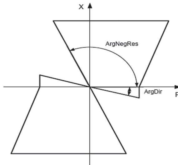
Figura 2. Selección de direccionalidad de la función de impedancia.
