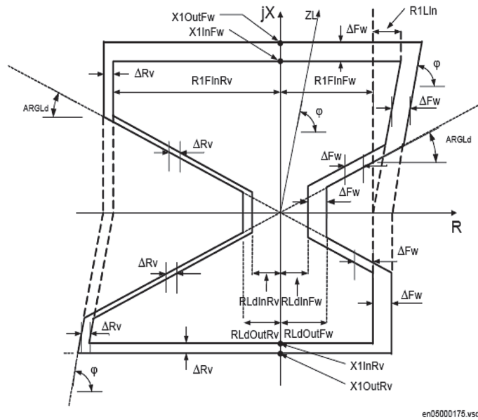
Figura 7. Característica de operación de la detección de oscilación de potencia.
