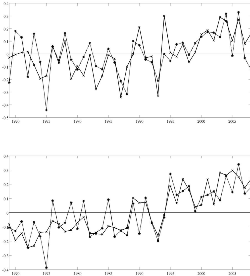
Figura 7. Series de tiempo normalizadas para los segundos modos en los modelos: a) AMP, b) DCP, c) P80 y d) P10. En todas se utilizó la TSM de julio como predictor. Las líneas continuas con cruces son las series de tiempo anuales de la TSM, mientras que las líneas a trazos con asteriscos representan el modo de la variable estadística correspondiente para el trimestre ASO. El periodo base es de 1969 al 2008. La correlación canónica de estos modos fue de alrededor 0.9, 0.9, 0.8 y 0.6, respectivamente, con significación estadística entre el 90%-95% para AMP y P10 y por encima del 99% para DCP y P80, según Davis (1976).
