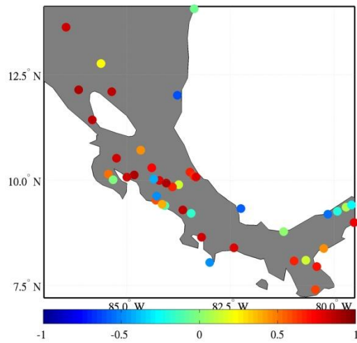
Figura 5. Pesos espaciales de los primeros modos de los predictantes de cada modelo: a) AMP, b) DCP, d) P80 y d) P10 para el trimestre ASO.
