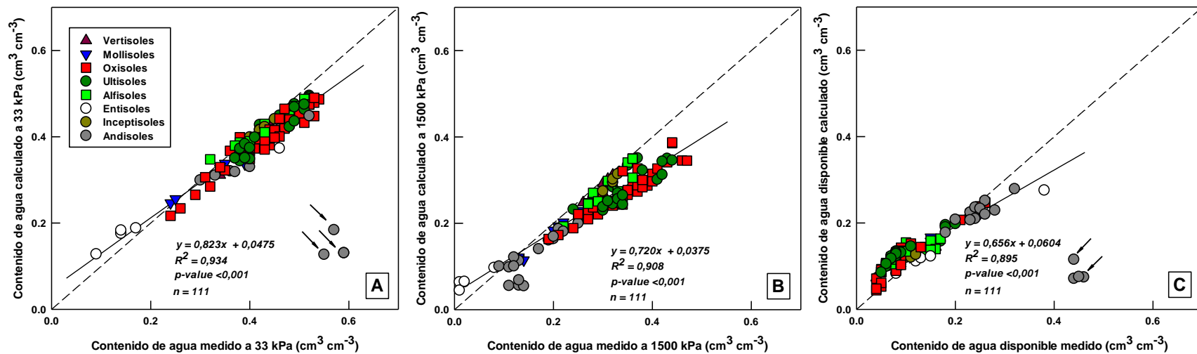
Figura 3. Comparación entre los resultados obtenidos de las funciones de pedotransferencia incluidas en el modelo Rosetta3 y los valores correspondientes obtenidos de los análisis de laboratorio para los contenidos de humedad de órdenes de suelos de Costa Rica: A) determinados a 33 kPa (CC); B) determinados a 1500 kPa (PMP), y C) el contenido de agua disponible del suelo (AD). Líneas discontinuas representan una relación 1:1 de los ejes del gráfico. Línea negra continua representa el modelo de mejor ajuste ( y = \beta_1 x + \beta_0 ) entre las variables. Flechas negras señalan valores atípicos, los cuales no se incluyeron en los análisis de regresión.
