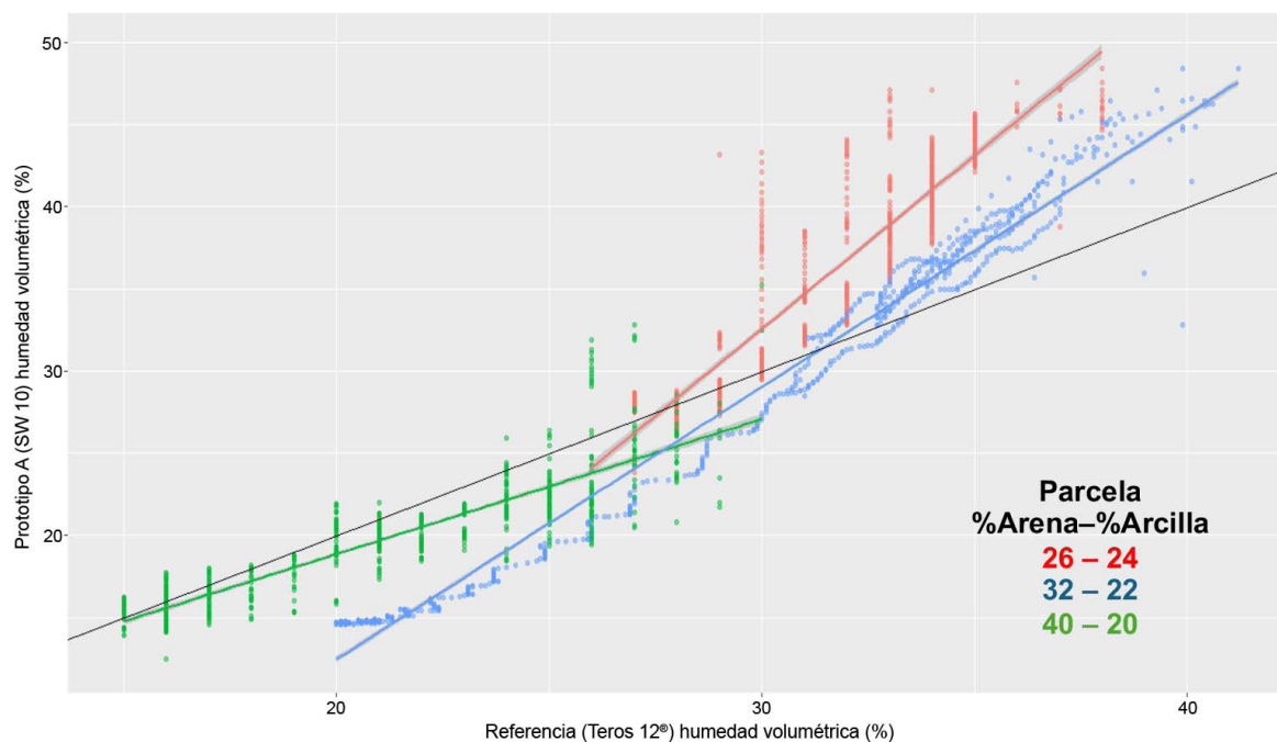
Figura 3. Regresiones por tipo de suelo de sensores de medición y registro de humedad de suelo, en parcelas La Vega, Zamorano, Honduras, enero de 2022.
