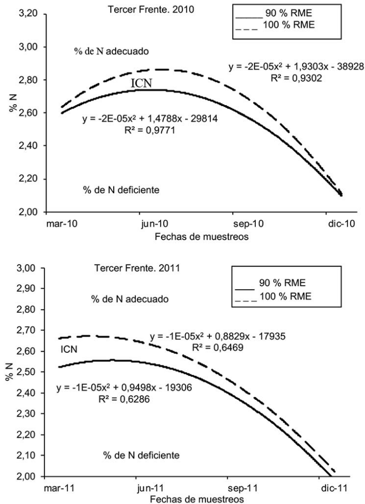
Figura 4. Intervalo crítico de nitrógeno para el C. canephora en la localidad de Tercer Frente, provincia de Santiago de Cuba, Cuba. 2010-2011.
