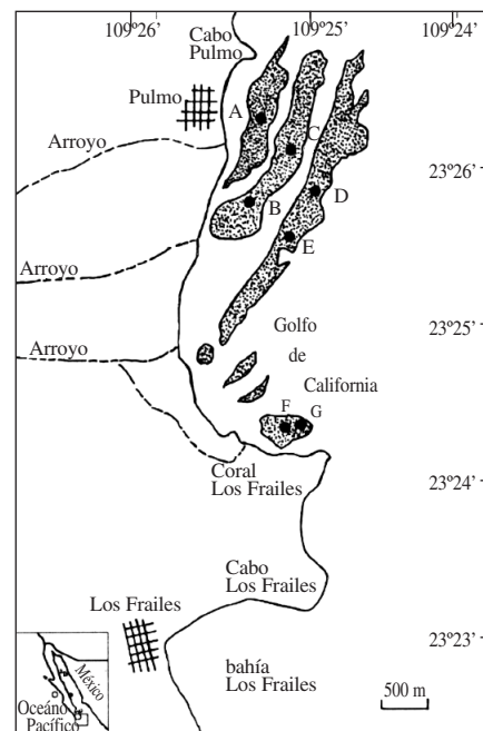
Fig. 1. Área de estudio. A) Primera barra (CP-588), B) segunda barra (CP-589-2), C) segunda barra (CP-989-2), D) tercera barra (CP-589-1), E) tercera barra (CP-989-1), F) Coral Los Frailes (CP-988), y G) Coral Los Frailes (CP-989-3).
