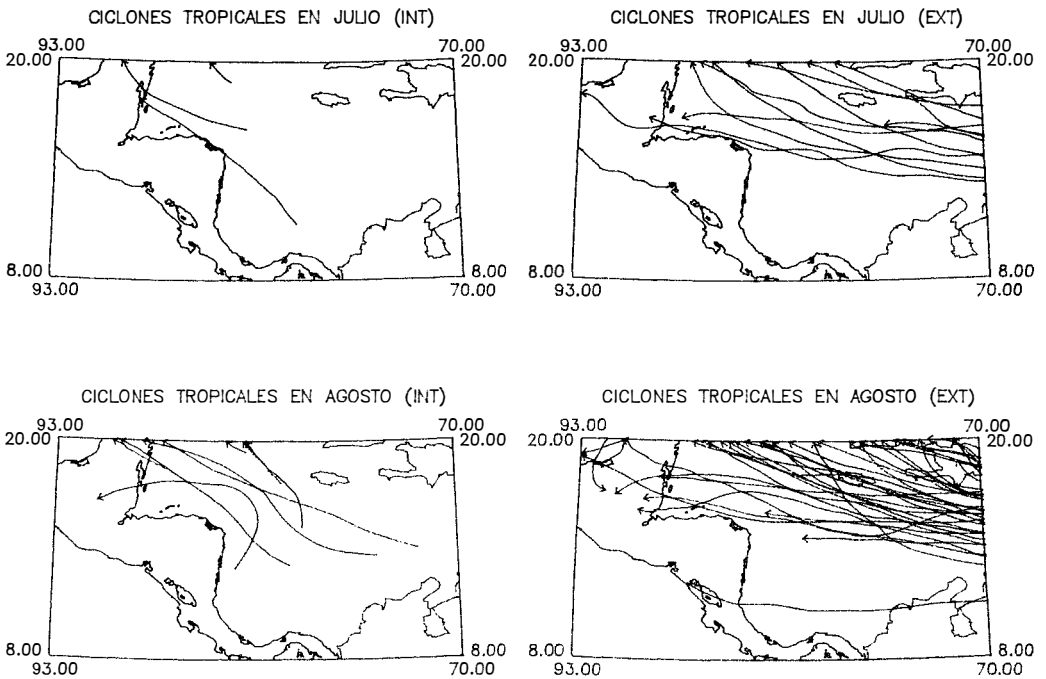
Fig. 4. Comparación entre las dos categorías de ciclones tropicales: Int./Ext., en función de los meses julio y agosto.
