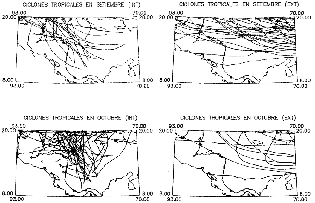
Fig. 5. Comparación entre las dos categorías de ciclones tropicales: Int./Ext., en función de los meses setiembre y octubre.
