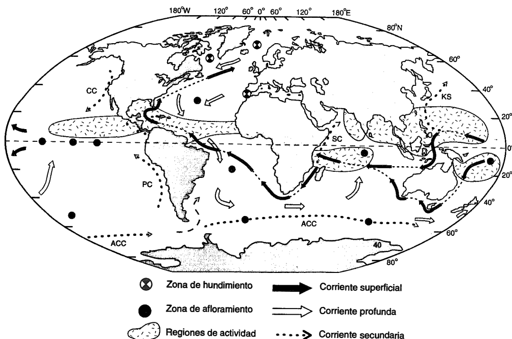
Fig. 2. Representación a nivel mundial del movimiento de las corrientes superficiales, de profundidad, y otras. Las regiones occidentales de los océanos describen zonas donde se da la gestación de ciclones tropicales, a ambos lados del Ecuador.
