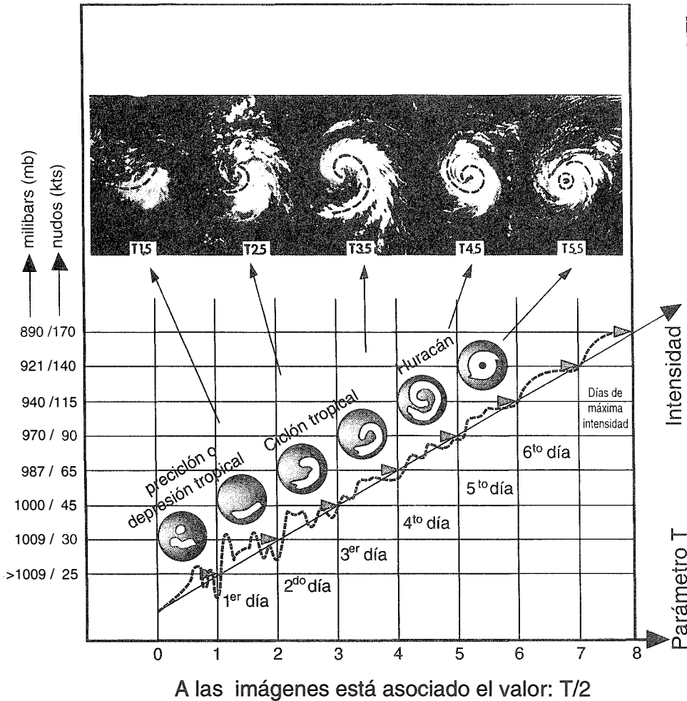
Fig. 7. En función de la presión en el centro del fenómeno, la velocidad de los vientos sostenidos, y del parámetro T, al cual se asocia el tiempo de maduración, se presentan las posibles fases de una depresión tropical, siendo la de un huracán maduro una conformación compacta: con T5.5 (Adaptado de Dvorak y Smigielski 1996).
