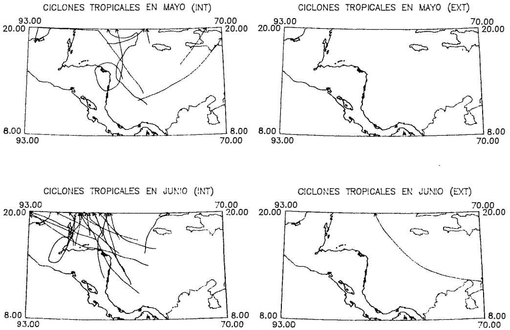
Fig. 3. Comparación entre las dos categorías de ciclones tropicales: Int./Ext., en función de los meses mayo y junio.
