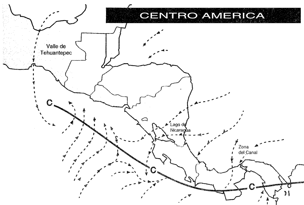
Fig. 1. Representación esquemática de los pasos de vientos que se dan en superficie sin ser perturbados fuertemente por la orografía. También se dan las posibles regiones donde se localizan los afloramientos costeros en la región oriental del Pacífico (Adaptado de Guard 1986).
