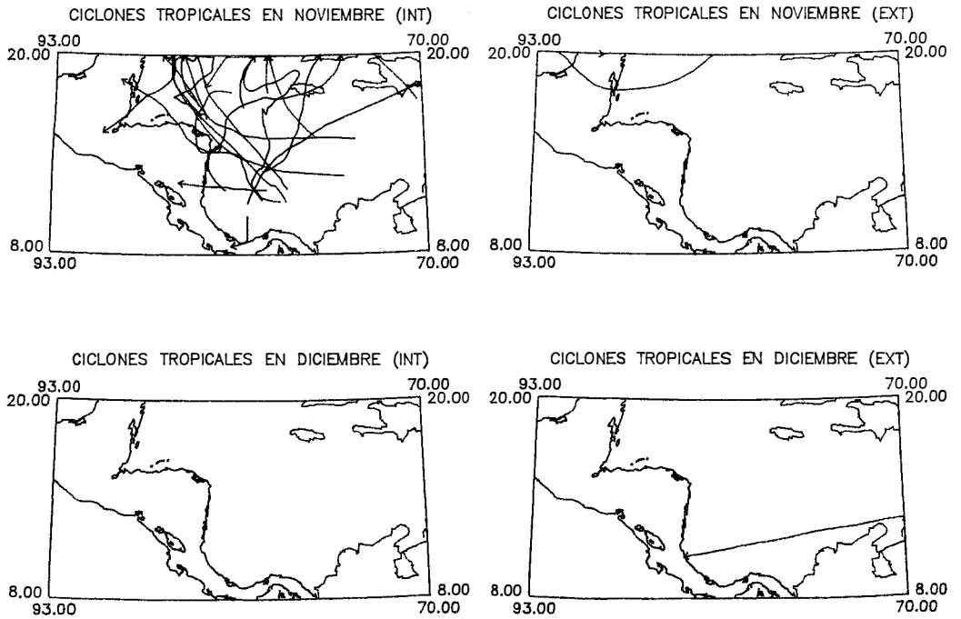
Fig. 6. Comparación entre las dos categorías de ciclones tropicales: Int./Ext., en función de los meses noviembre y diciembre.
