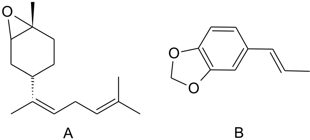
Fig. 1. Estructuras químicas del epóxido trans-Z- \alpha -bisaboleno (A) y del Safrol (B) aislados del fruto inmaduro y maduro de P. auritum .
