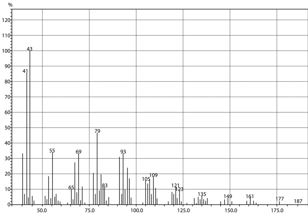
Fig. 2. Espectro de masas del trans-Z- \alpha -bisaboleno epóxido.
