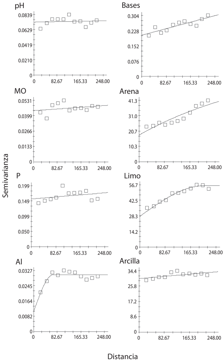
Fig. 4. Variogramas isotrópicos de las variables edáficas en una parcela de 6ha (120x500m) en el PNNA usando la BD-1. El eje de las abcisas representa la distancia en metros y el eje de las ordenadas representa la semivarianza. pH: modelo lineal. MO: modelo lineal. P: modelo lineal. Al: modelo esférico. Bases: modelo lineal. Arena: modelo exponencial. Limo: modelo esférico. Arcilla: modelo lineal.
