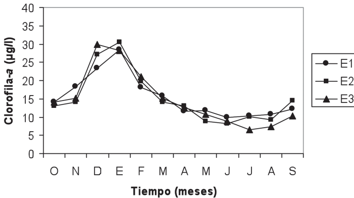
Fig. 4. Variación de la biomasa del fitoplancton (concentración de clorofila a) en las tres estaciones de muestreo durante el periodo de estudio.
