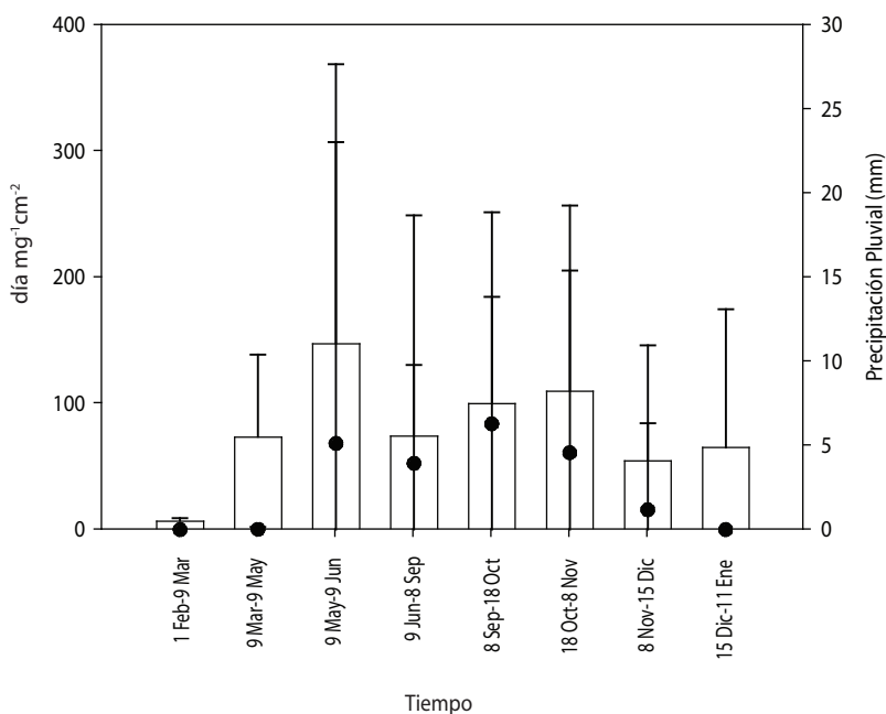
Fig. 2. Tasa de sedimentación ( \text{mg cm}^{-2} \text{ día}^{-1} ) y precipitación pluvial media (mm) en Bahías de Huatulco durante un ciclo anual (febrero 2006-enero 2007). Barras = tasa de sedimentación, círculos = precipitación pluvial media.
