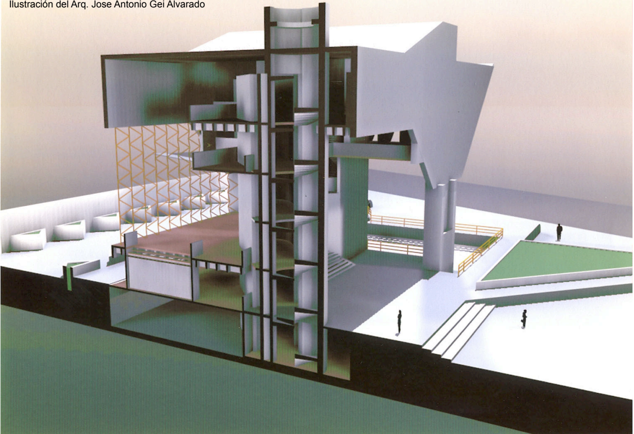
Sección de norte a sur. Ilustración del Arq. Jose Antonio Gei Alvarado
