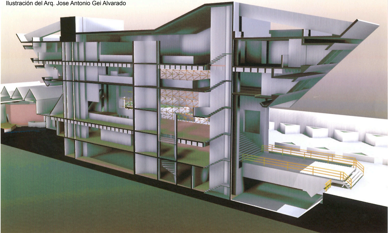
Sección de norte a sur. Ilustración del Arq. Jose Antonio Gei Alvarado
