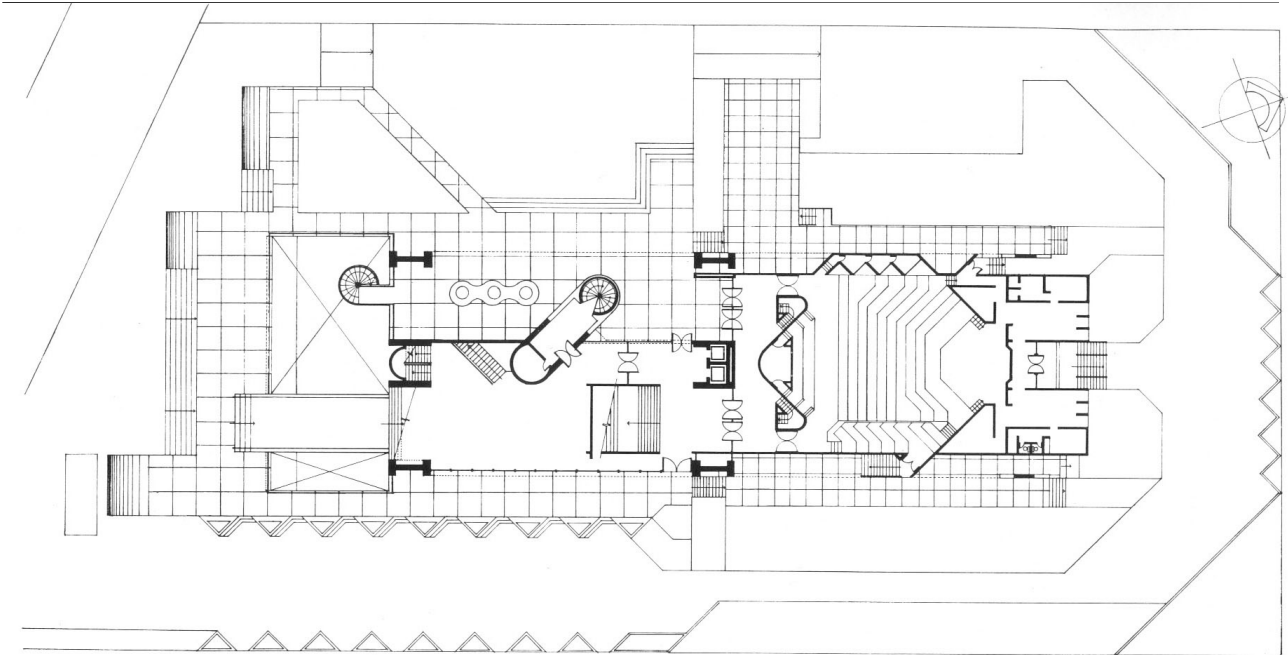
Planta arquitectónica del primer nivel. Dibujo propiedad del Arq. Hernán Jiménez
