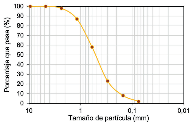
Figura 3. Curva granulométrica de la arena residual
