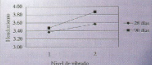
Gráfico 9. Hendimiento vs Nivel de vibrado según edad para testigos ensayados al nivel de humedad 3
