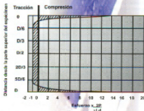
Figura 2. Distribución del esfuerzo horizontal en un cilindro cargado.
