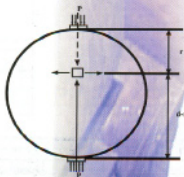
Figura 1. Prueba brasileña de tracción.
