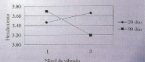
Gráfico 8. Hendimiento vs Nivel de vibrado según edad para testigos ensayados al nivel de humedad 2
