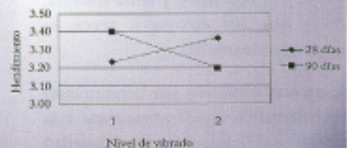
Gráfico 7. Hendimiento vs Nivel de vibrado según edad para testigos ensayados al nivel de humedad 1
