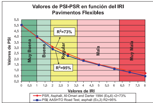
Gráfico 1 Rangos de IRI para pavimentos flexibles. Modelo de correlación con PSI
