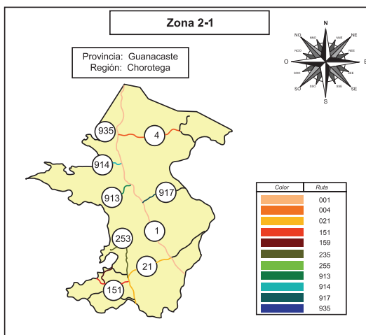
Figura 3 Determinación de los tramos homogéneos, valores de IRI y PSI para la zona 2-1 de Conservación Vial, Costa Rica 2008
