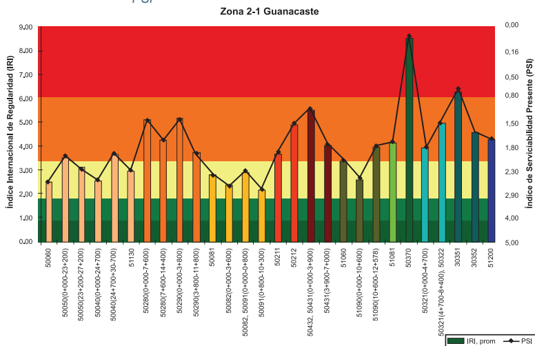
Gráfico 2 Rangos de IRI para pavimentos flexibles. Modelo de correlación con PSI
